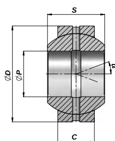
TYPE FO
